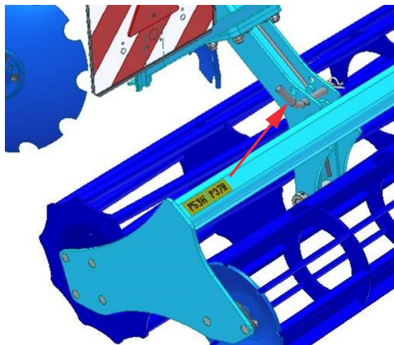
Obr. 5 - zadní dvojitý válec v převravní poloze
