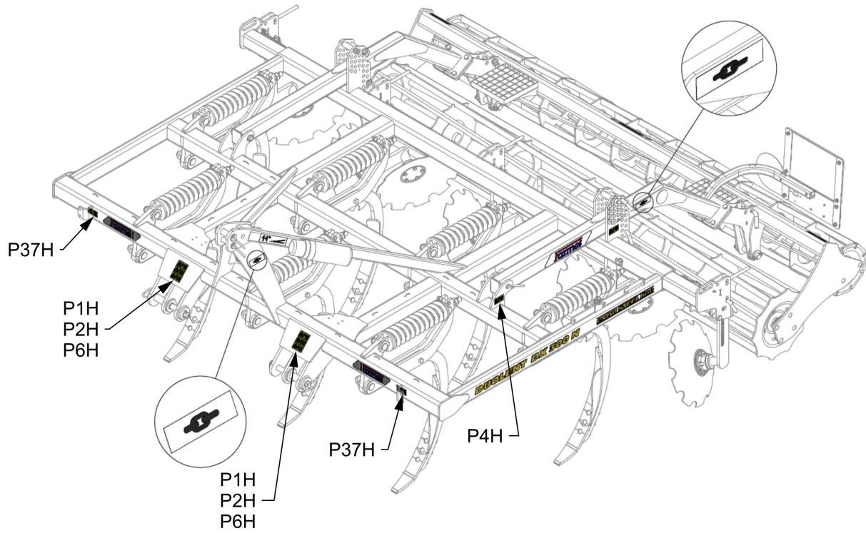
Obr. 1 - Umístění bezpečnostních štítků na stroji
