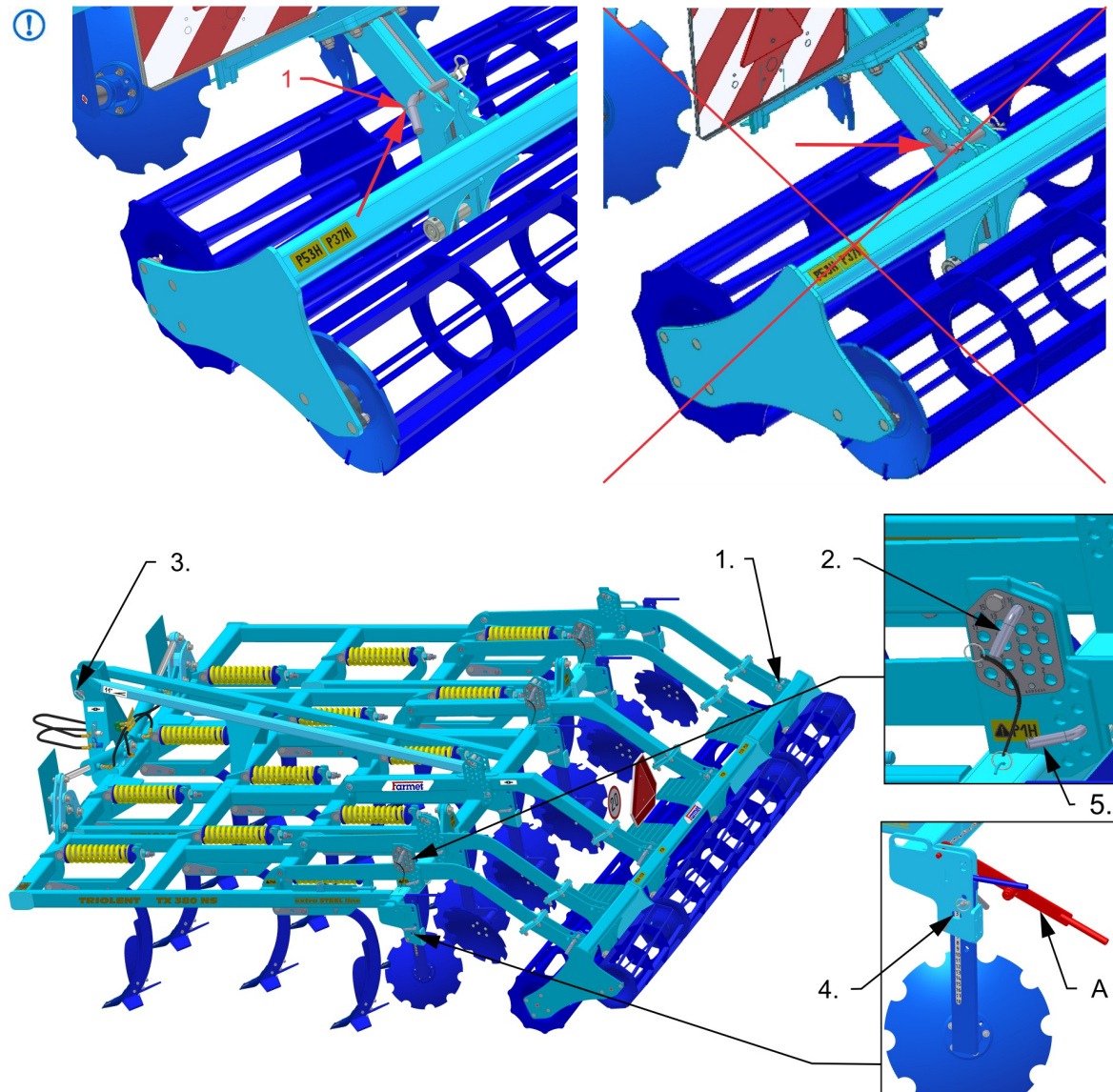
Obr. 8 - postup seřízení stroje
