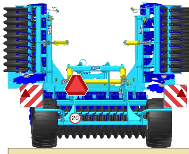
Zum Auseinanderklappen vorbereitete Maschine
