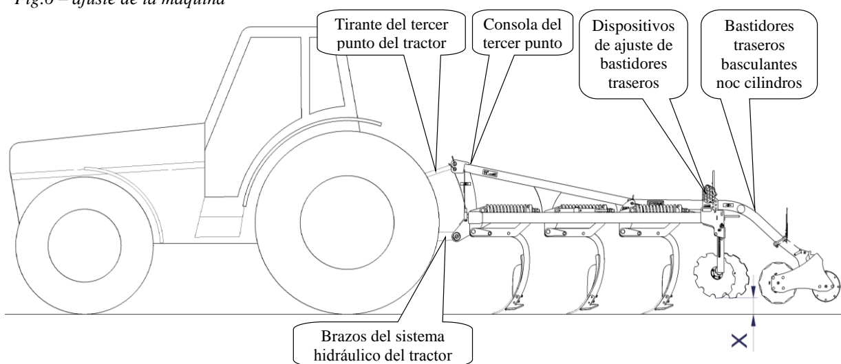
Fig.6 – ajuste de la máquina
