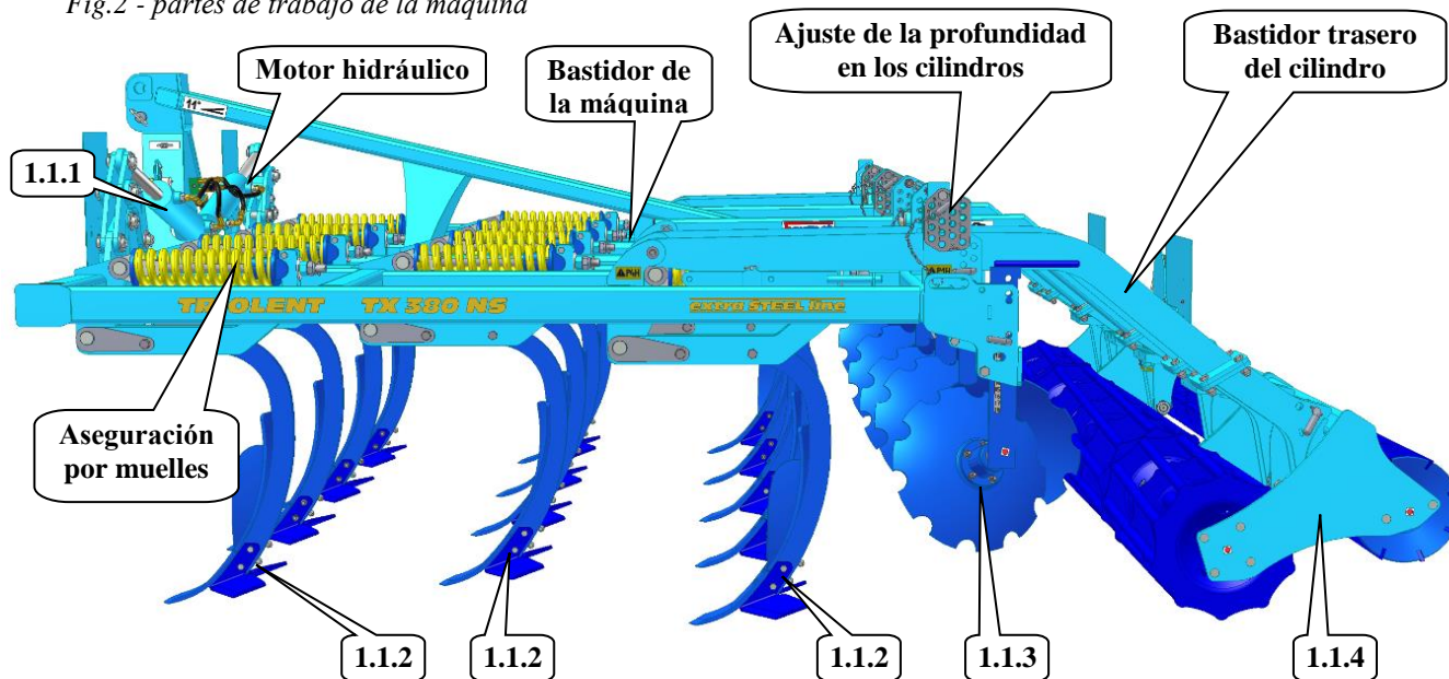
Fig.2 - partes de trabajo de la máquina
