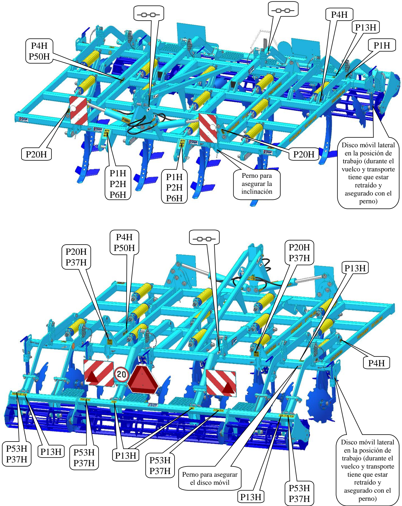
Fig.1-Colocación de las etiquetas de seguridad en la máquina
