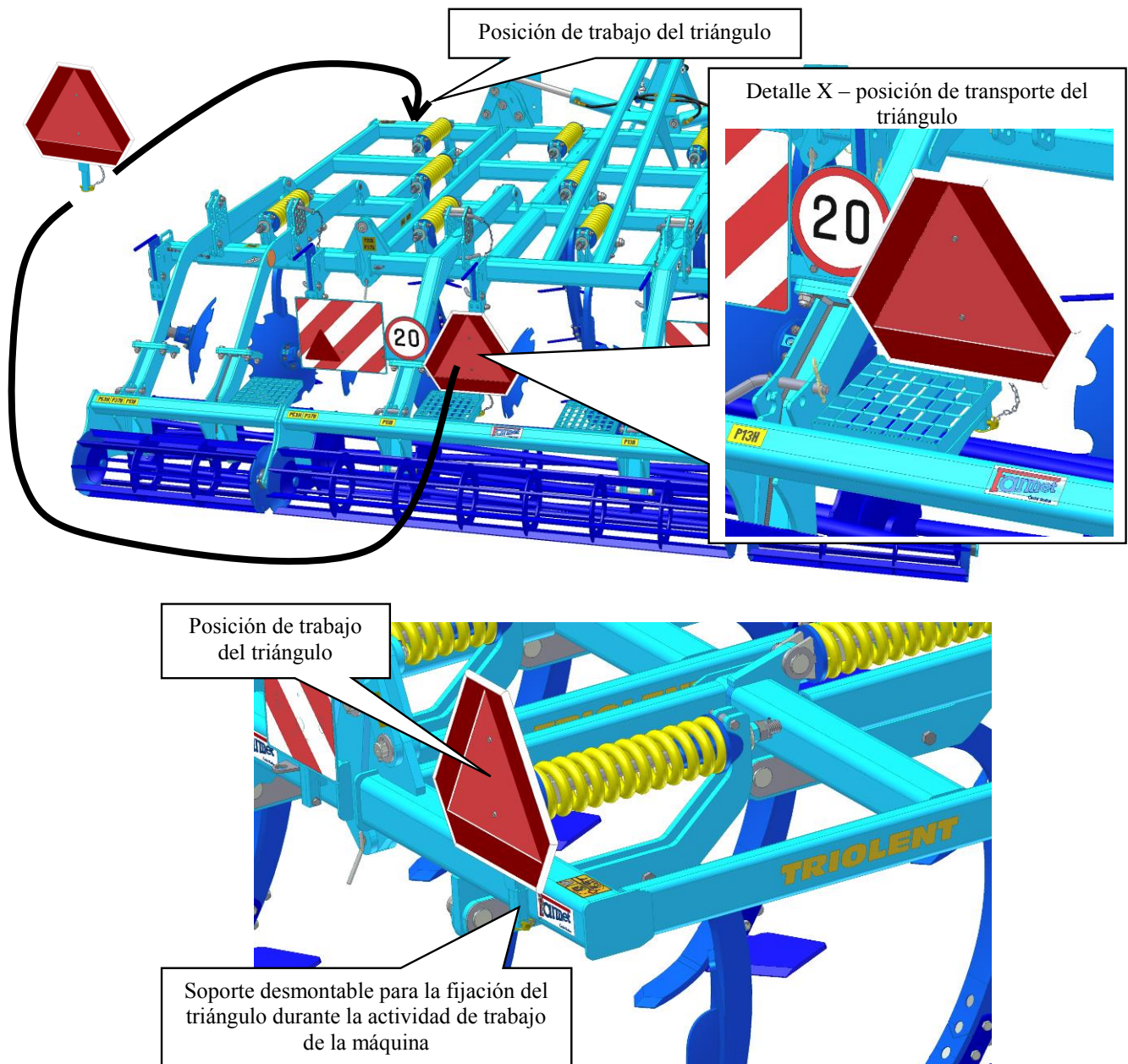
Fig.5 – colocación del triángulo de marca trasera de vehículos lentos
