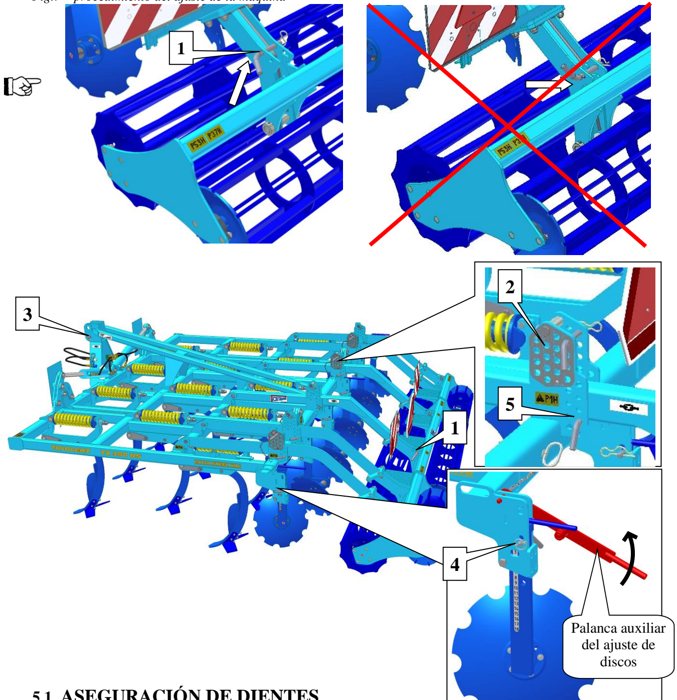
Fig.7 – procedimiento del ajuste de la máquina
