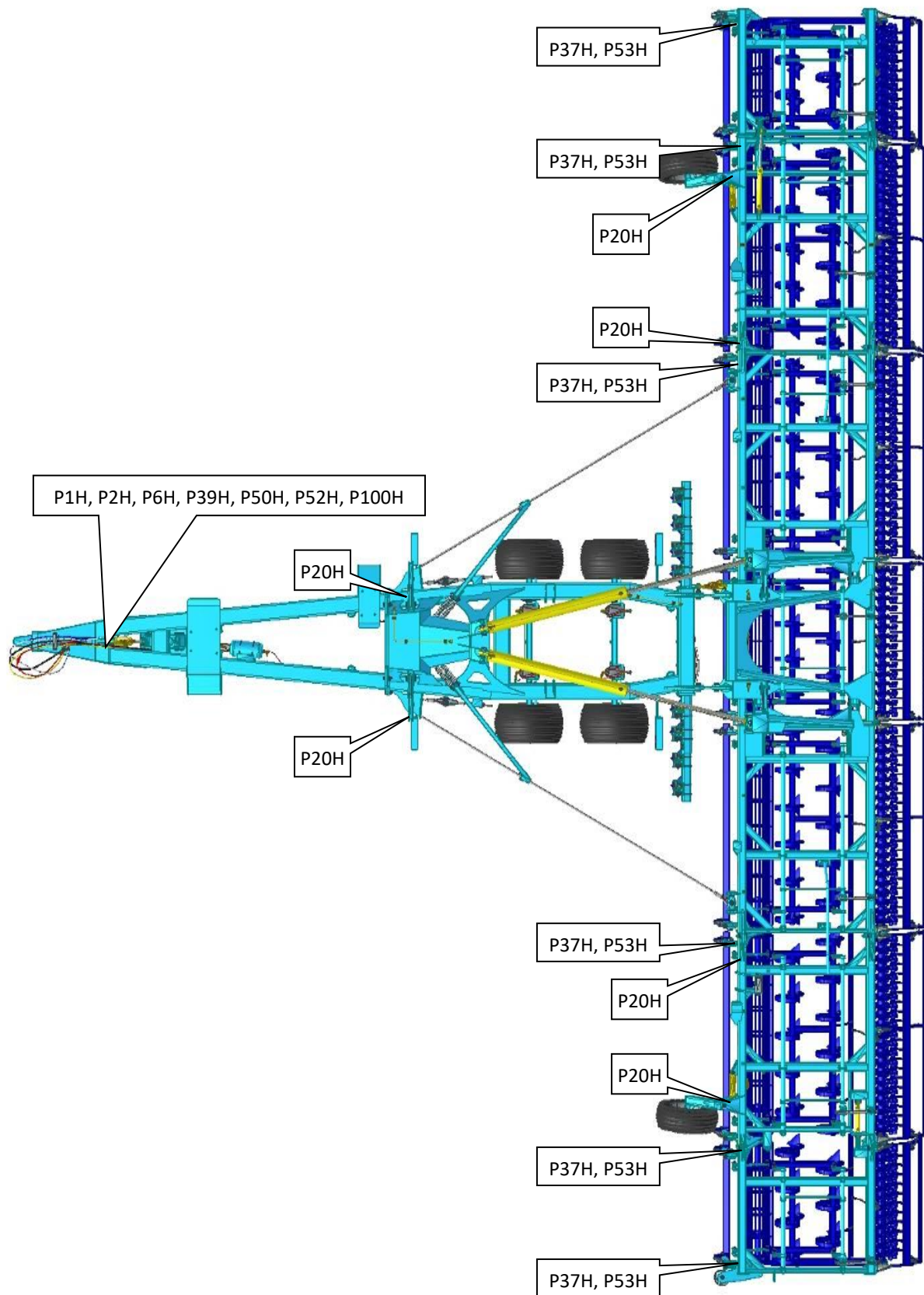
рис. 1 - расположение самоклеющихся предохранительных табличек на K 1250 PS, K 1570 PS
