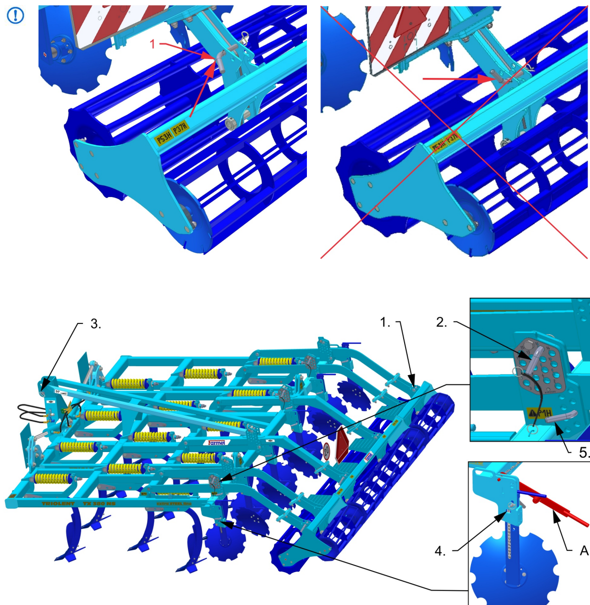
Rys. 7 - sposób postępowania podczas ustawienia maszyny
