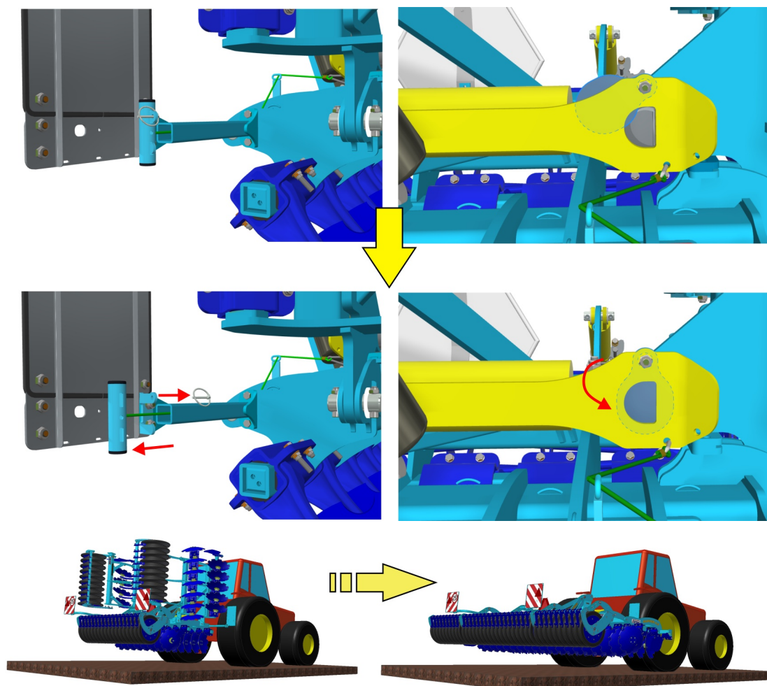
Rys. 2 - Odblokowanie ciągnika
