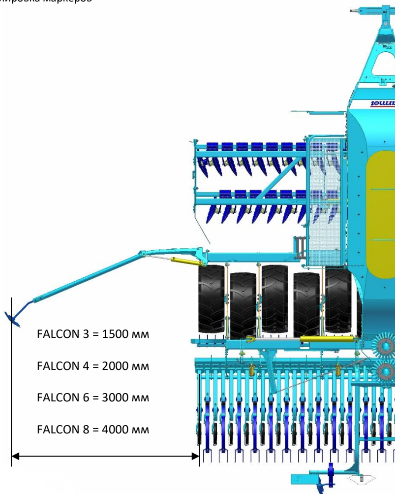
Рис. 62 - регулировка маркеров
