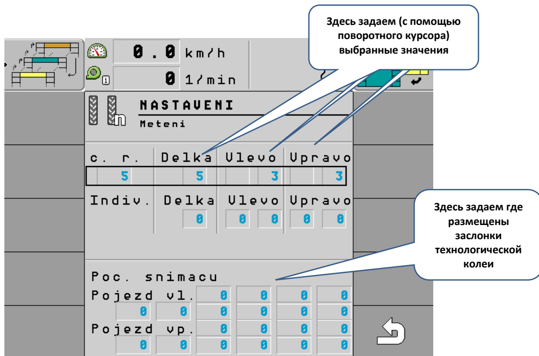
Рис. 19 – Установка ритма технологической колеи на блоке отображения
