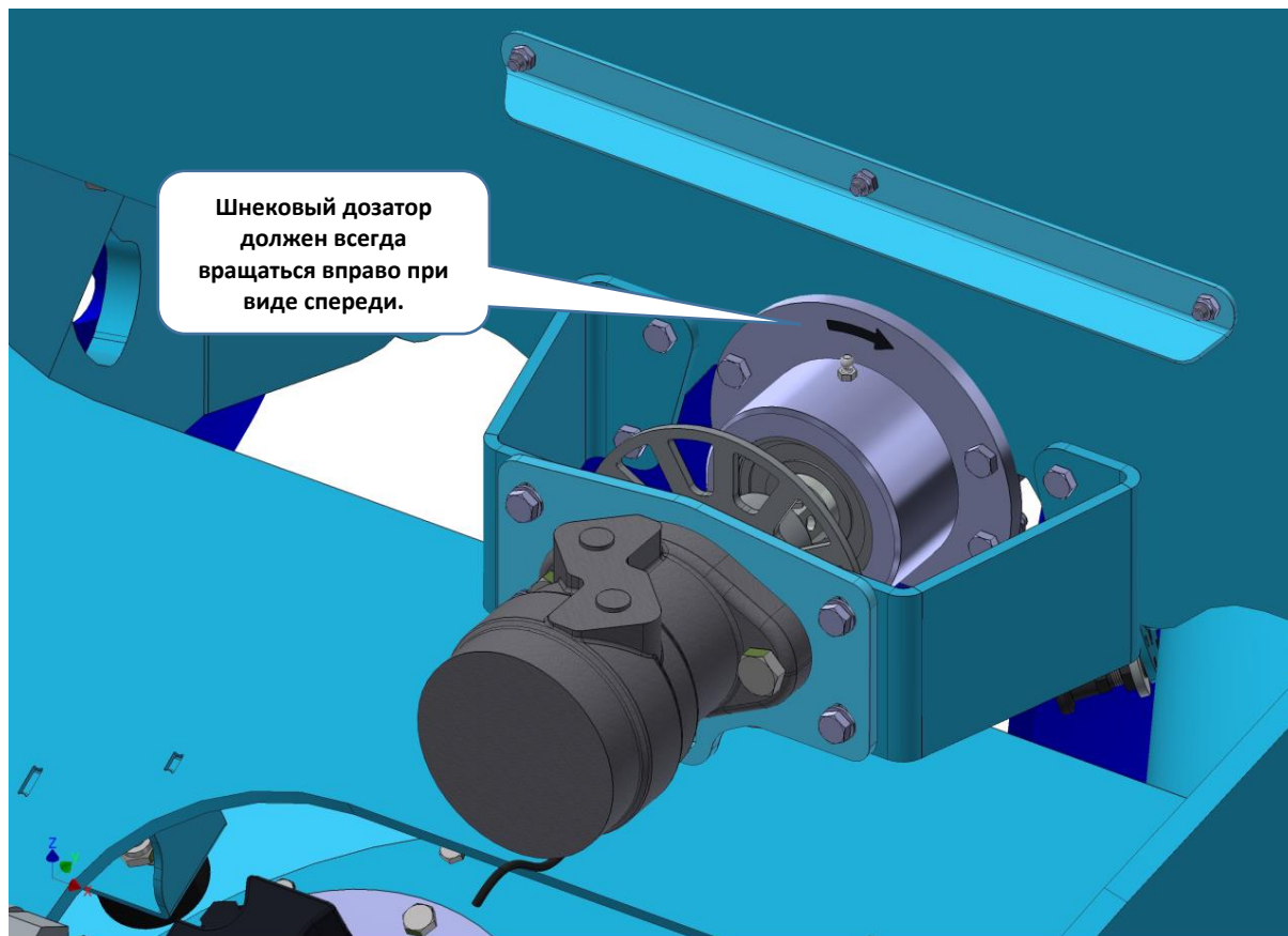
Рис. 40 - направление вращения дозатора внесения удобрений
