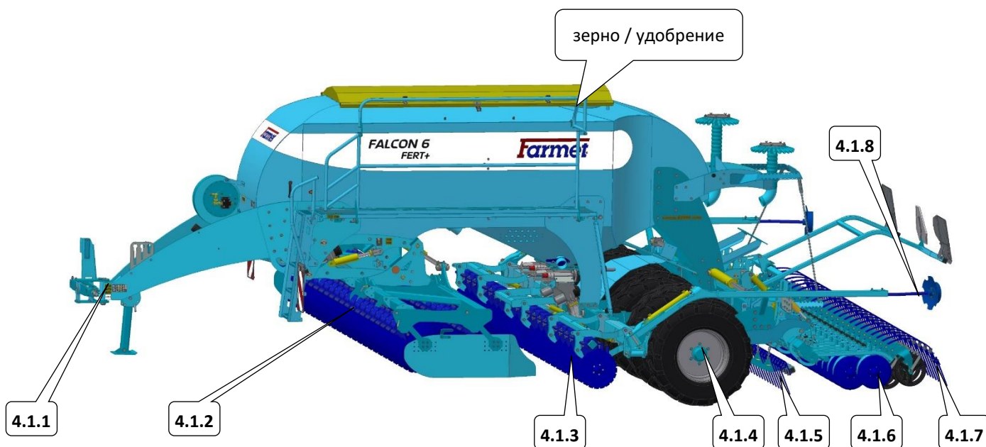
рис.3 - рабочие узлы машины
