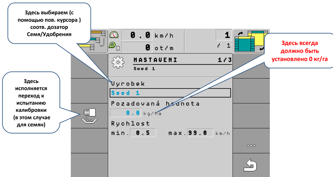
Рис. 43 - Установка дозировки высева для одного дозатора семян для дозировки 50 кг/га
