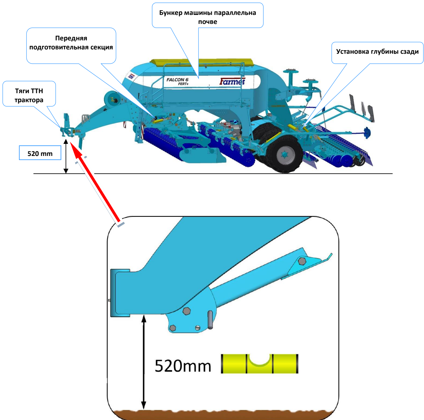
Рис. 55 - настройка ТТН
