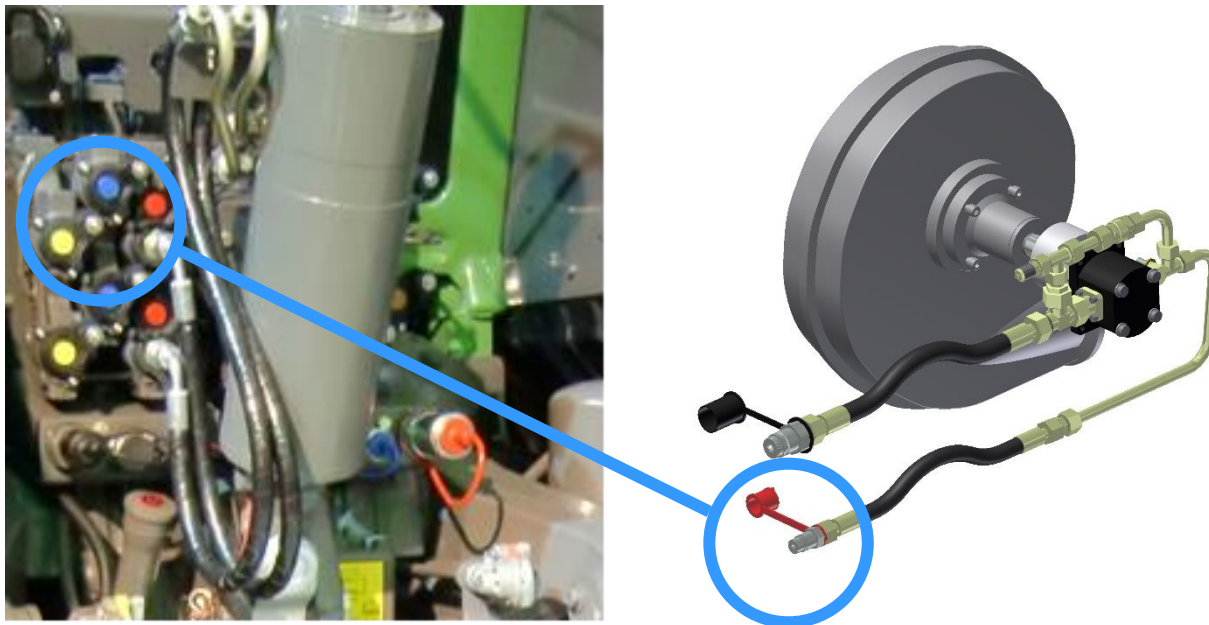
Рис 8 – подсоединение напорного шланга
