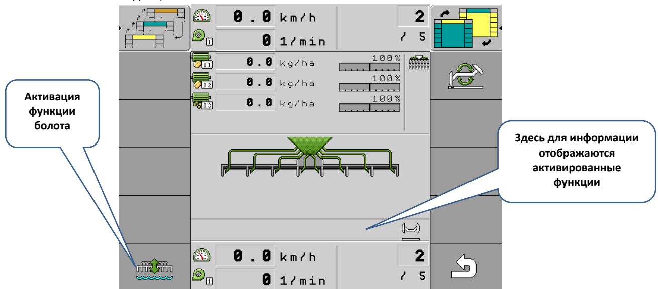
Рис. 16 – Описание функций
