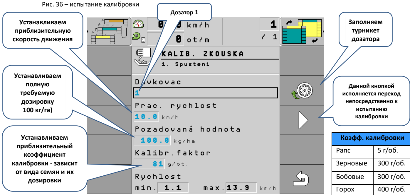
Рис. 36 – испытание калибровки
