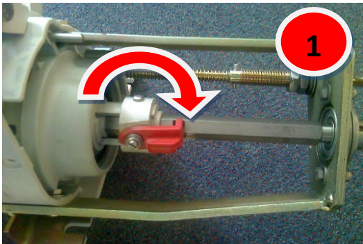
Рис. 41 – Настройка микровысева
