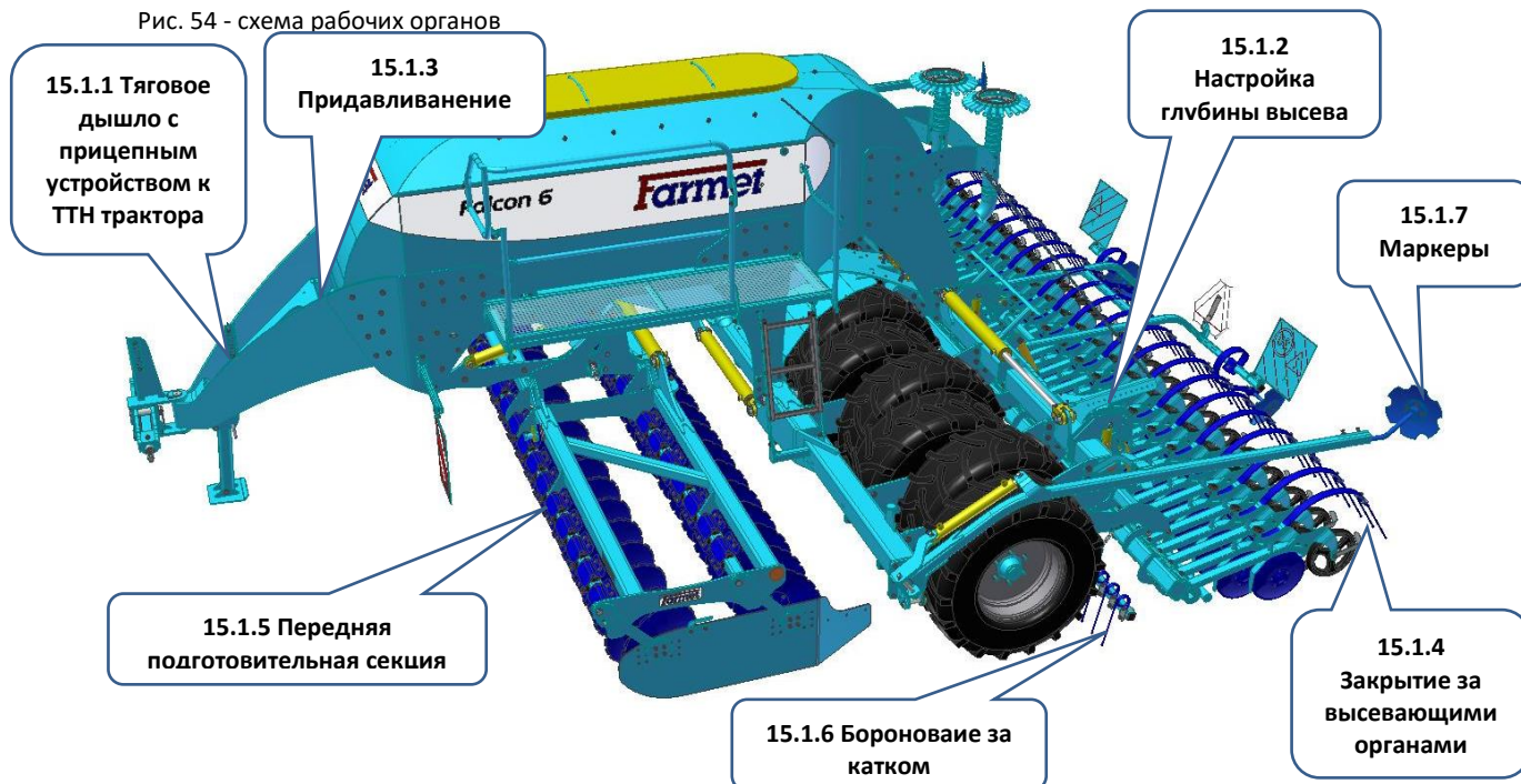
Рис. 54 - схема рабочих органов
