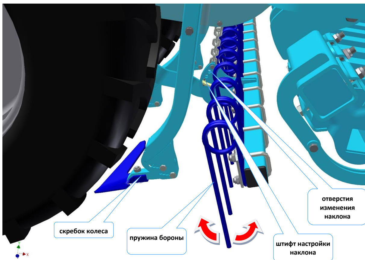
Рис. 61 - регулировка бороны
