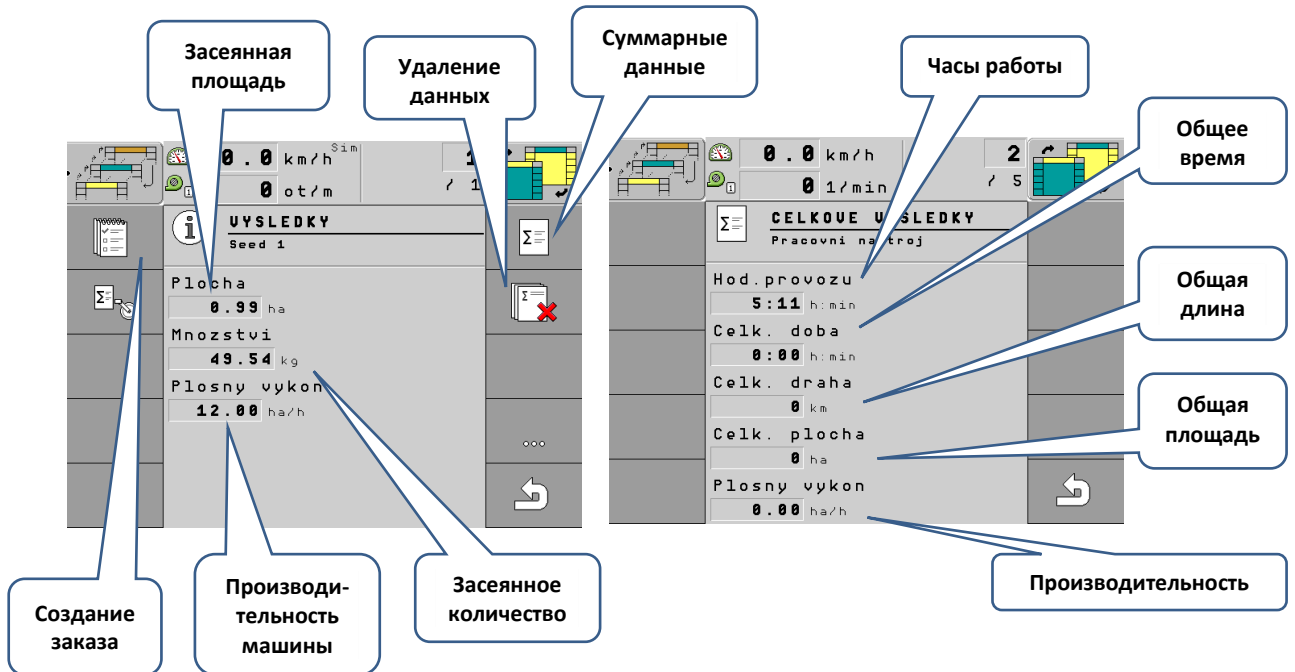
Рис. 20 - Информационные данные
