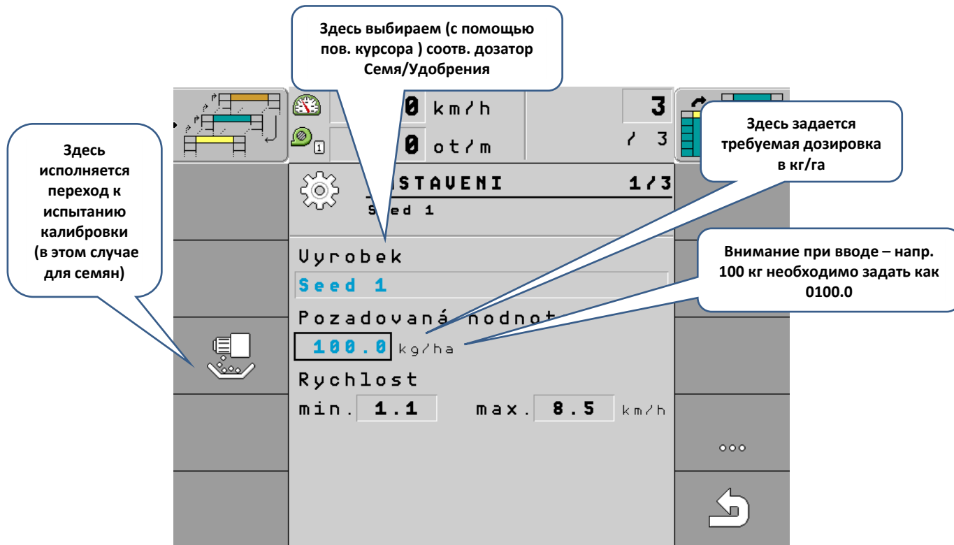
Рис. 35 - Установка одинаковой дозировки высева для двух дозаторов семян (100 кг/га оба дозатора одновременно)
